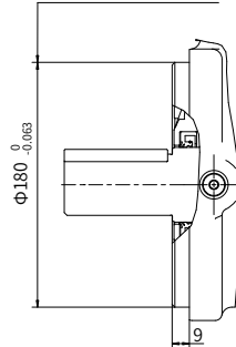
ISO 3019/2-180A2HW
