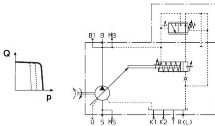
Схема регулятора давления DR
