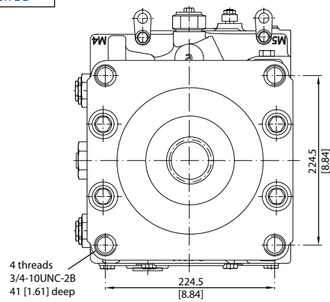
SAE E, option EG
